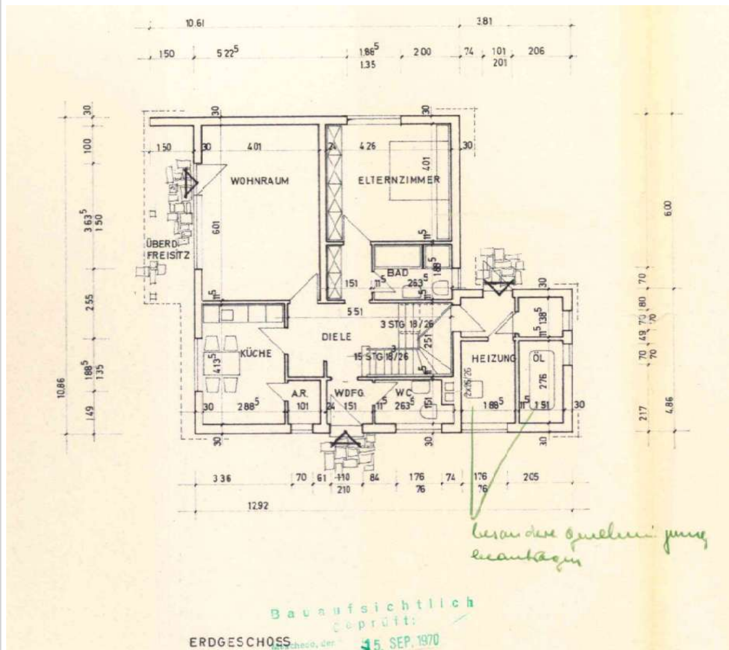
Grundriss Neubau
